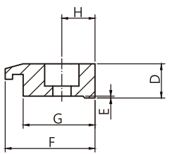
輔助視圖
